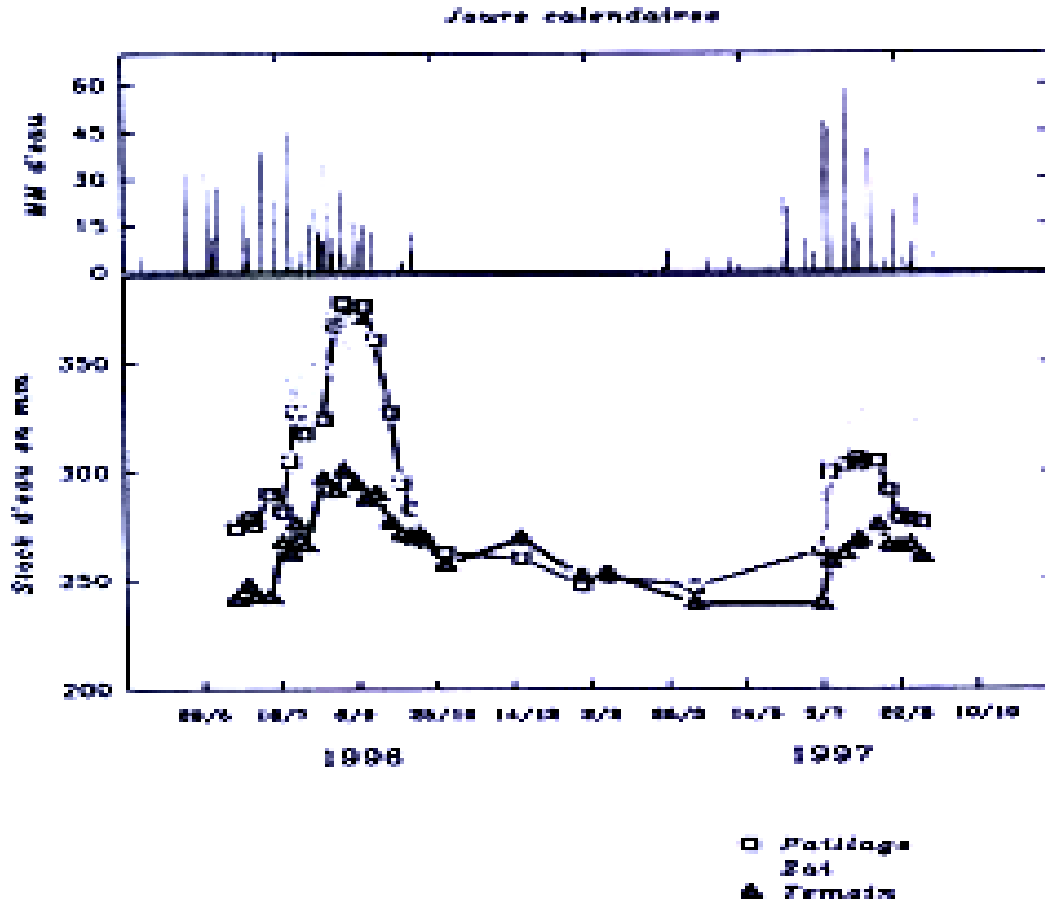
Figure n°2 : Effet de la pratique du paillage et du zai sur les variations des réserves en eau d'un sol encroûté en 1996 et 1997(Ambouta J.M.K., Moussa I.B. et Daouda O.S., 2000)
